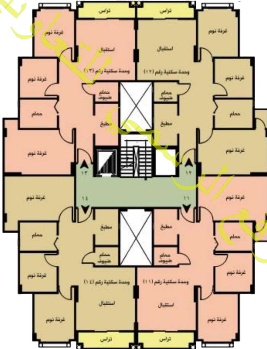
مسقط افقى للدور المتكرر
