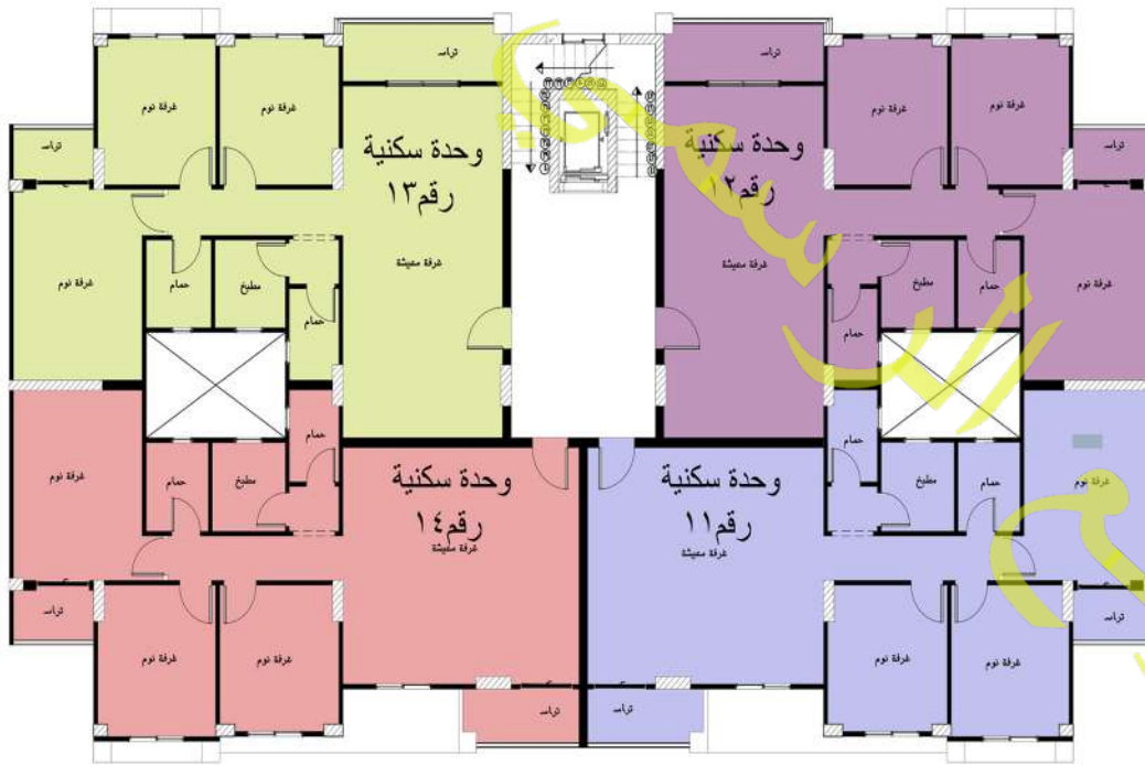
المسقط الافقي للدور المتكرر
